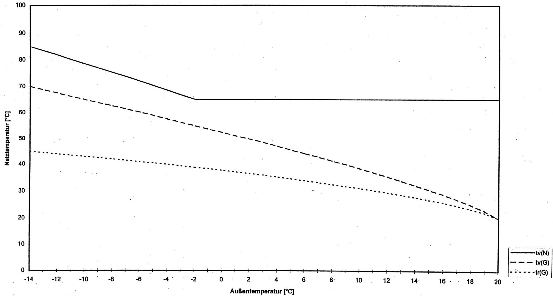
belzig_netztemperaturen Diagramm 2
