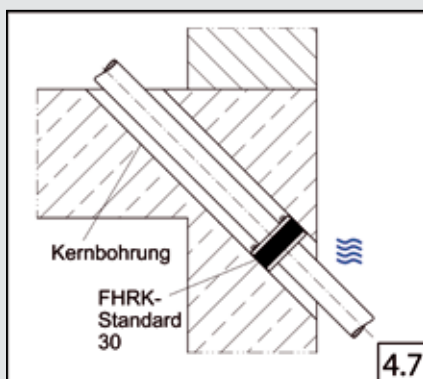
Bodeneinführung WU-Bodenplatte mit Kernbohrung
