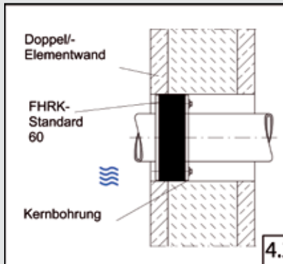
Wandeführung WU-Doppel-/ Elementwand mit Kernbohrung
