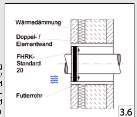
Wandeführung Doppel-/ Elementwand mit Wärme- dämmung und Futterrohr
