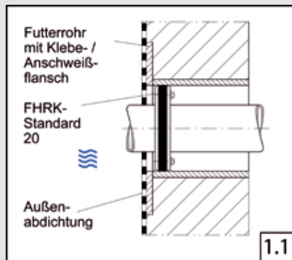
Wandeführung Mauerwerk-/ Betonwand mit Klebe-/ Anschweiß- flansch
