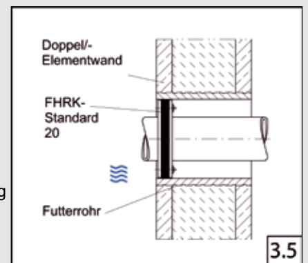
Wandeführung Doppel-/ Elementwand mit Futterrohr
