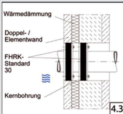
Wandeführung WU-Doppel-/ Elementwand mit Wärme- dämmung und Kernbohrung
