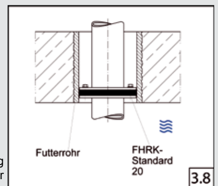
Bodeneinführung mit Futterrohr
