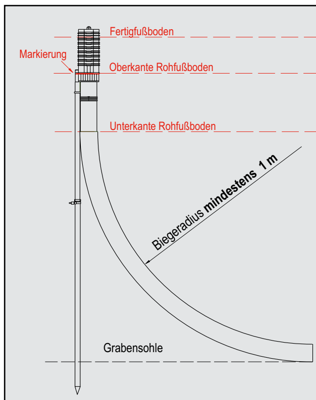
Mehrsparten-Hauseinführung
