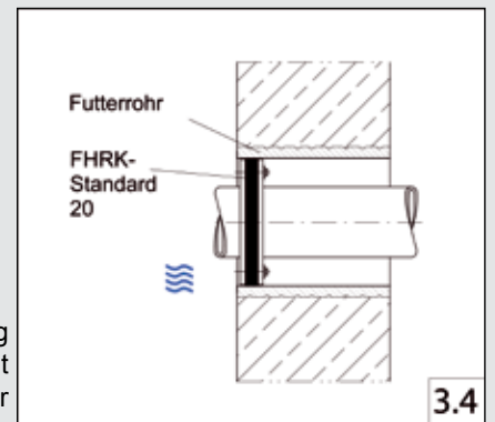
Wandeführung Betonwand mit Futterrohr
