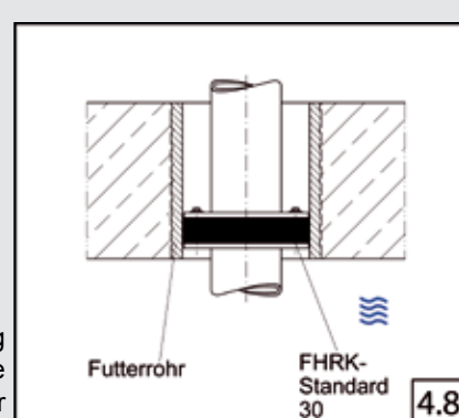
Bodeneinführung WU-Bodenplatte mit Futterrohr
