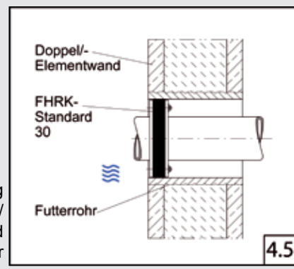
Wandeführung WU-Doppel-/ Elementwand mit Futterrohr
